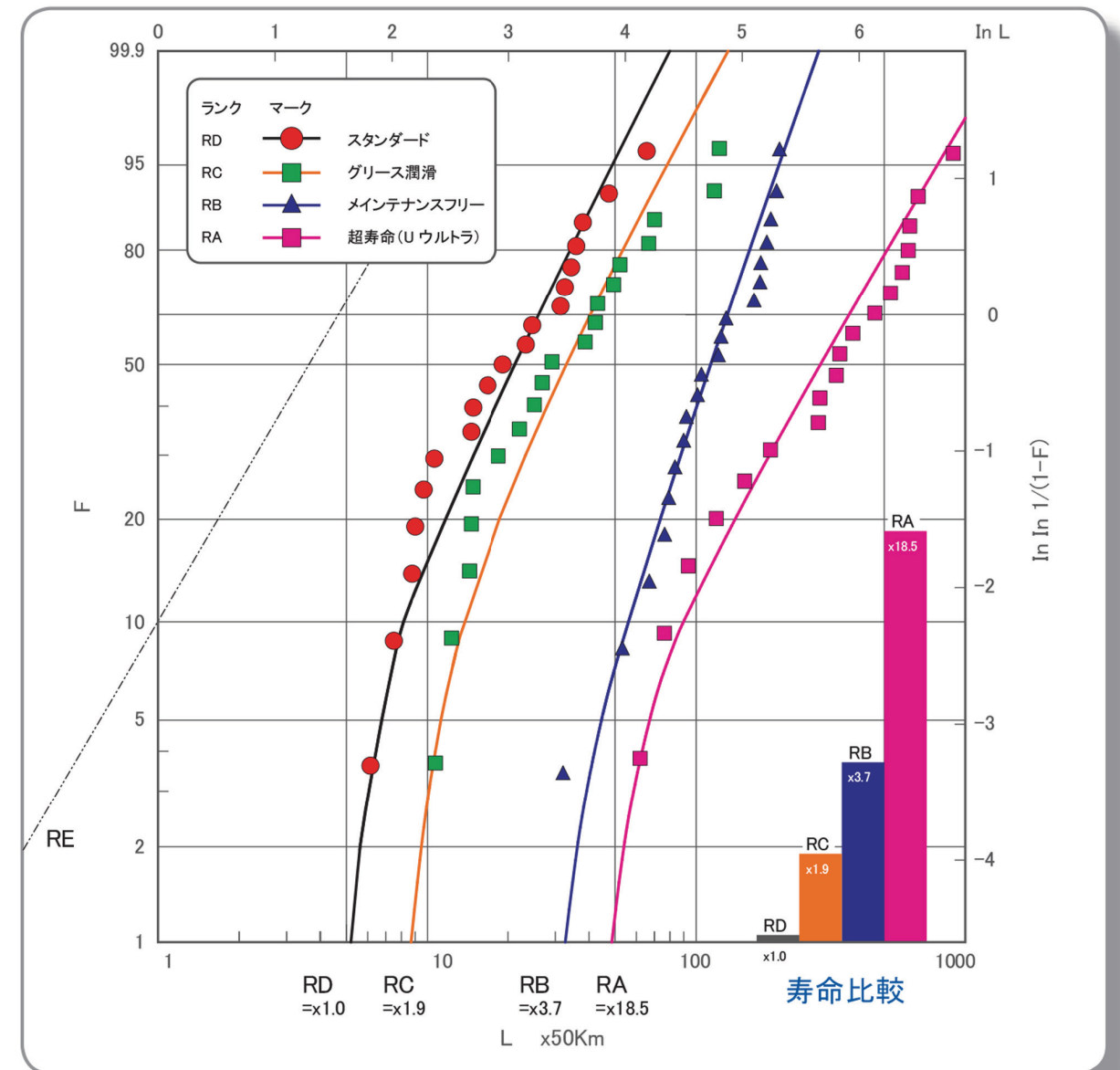
リニアベアリング信頼性設計ランク別選定基準 (RA~RD) と呼び番号
